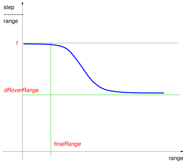
Fig. 7.1: Step limit.
