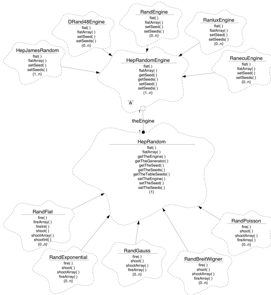
Fig. 2.24: HEPRandom module
